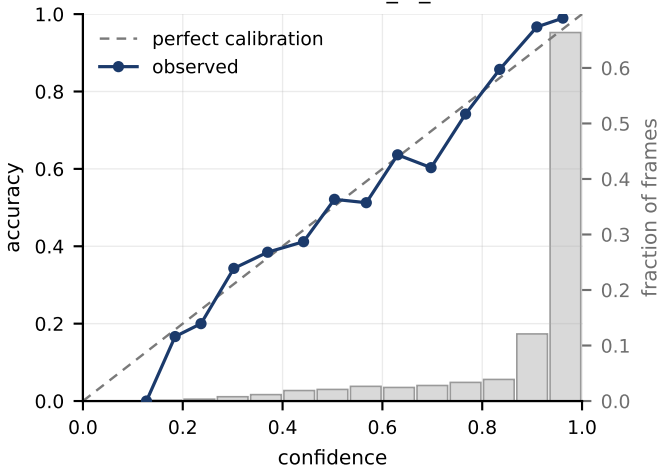
calibration — e1_rs_val
