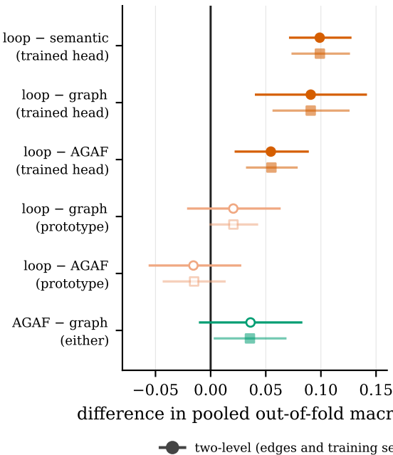
NF-UNSW-NB15
