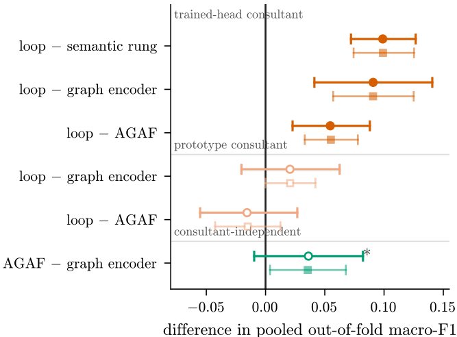
NF-UNSW-NB15
