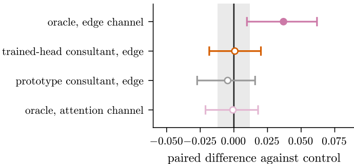
NF-UNSW-NB15
