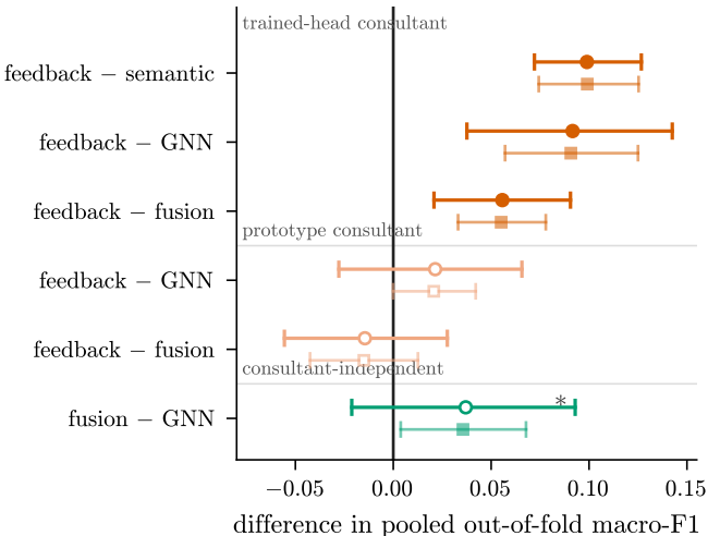
NF-UNSW-NB15
