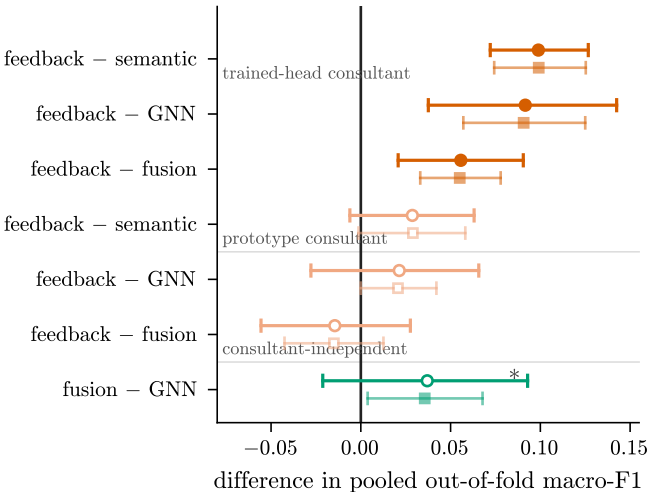
NF-UNSW-NB15
