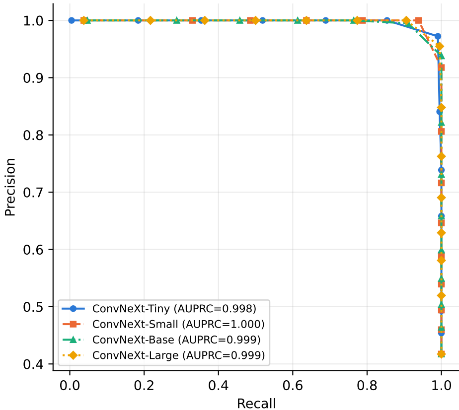
Kurva Precision-Recall -- test set (n=508)
