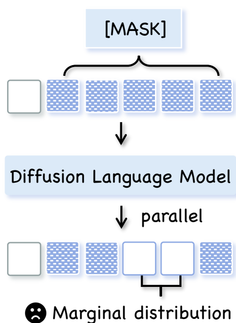
(d) MDLM
