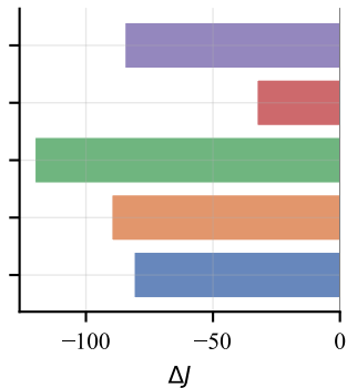
Param. Perturb.
