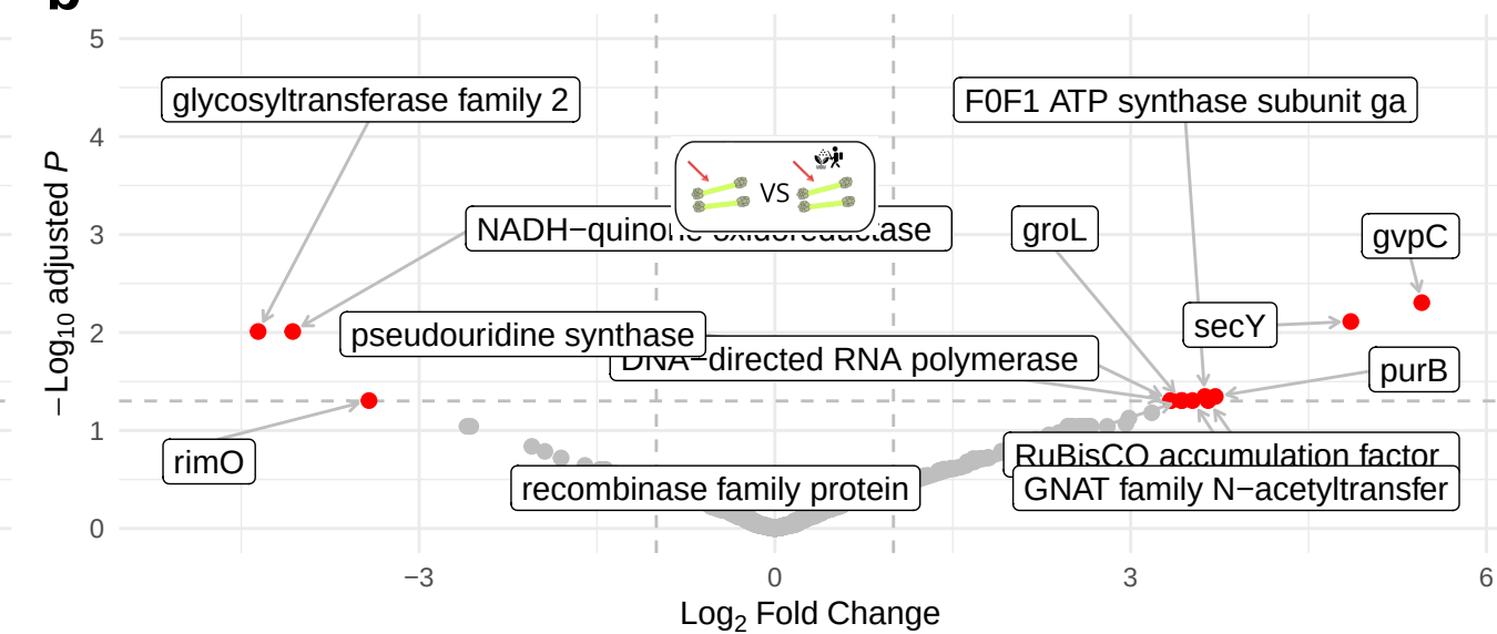
b infected cyanobacteria, no MET vs MET
