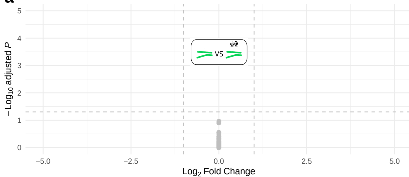
a free-living cyanobacteria, no MET vs MET
