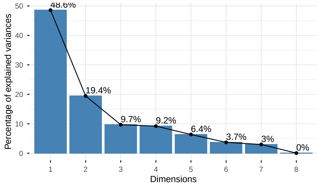
Varianza explicada por componente (SE3)
