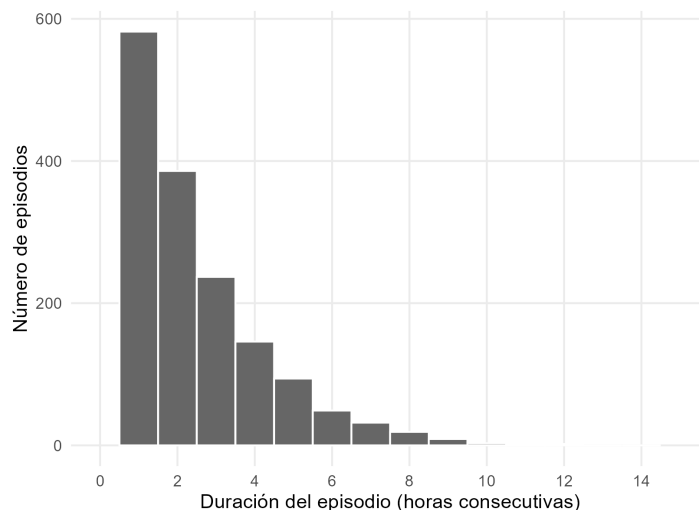
Figura 6: Distribución de la duración de los episodios de dióxido de azufre en SE3, medida en horas consecutivas por encima del umbral.
