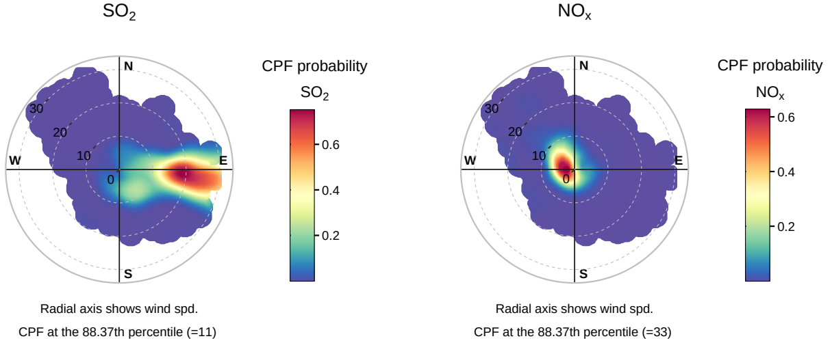
Figure 2: CBPF en SE3. Izquierda: SO_2 , con lóbulo direccional al este. Derecha: NO_x , con máximo central en condiciones de calma. Ambos paneles emplean el mismo percentil de referencia.
