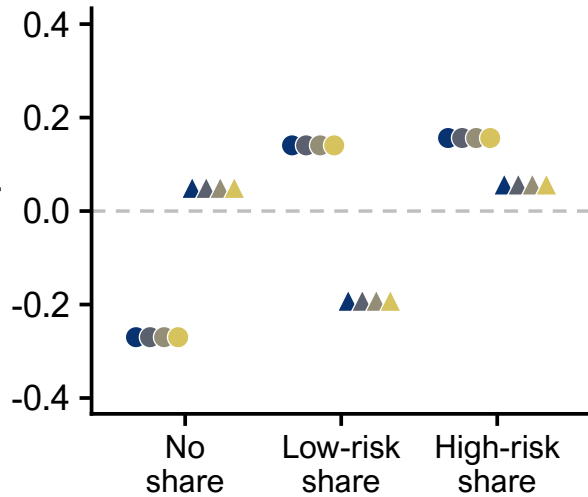
Belief update
