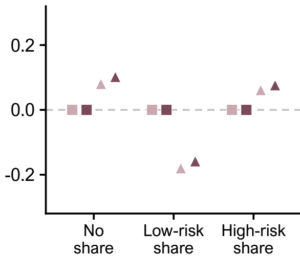
Belief update
