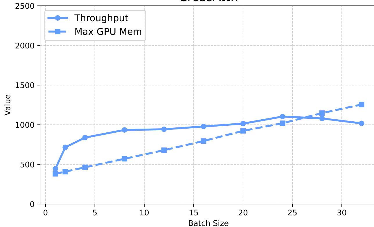
CrossAttn
