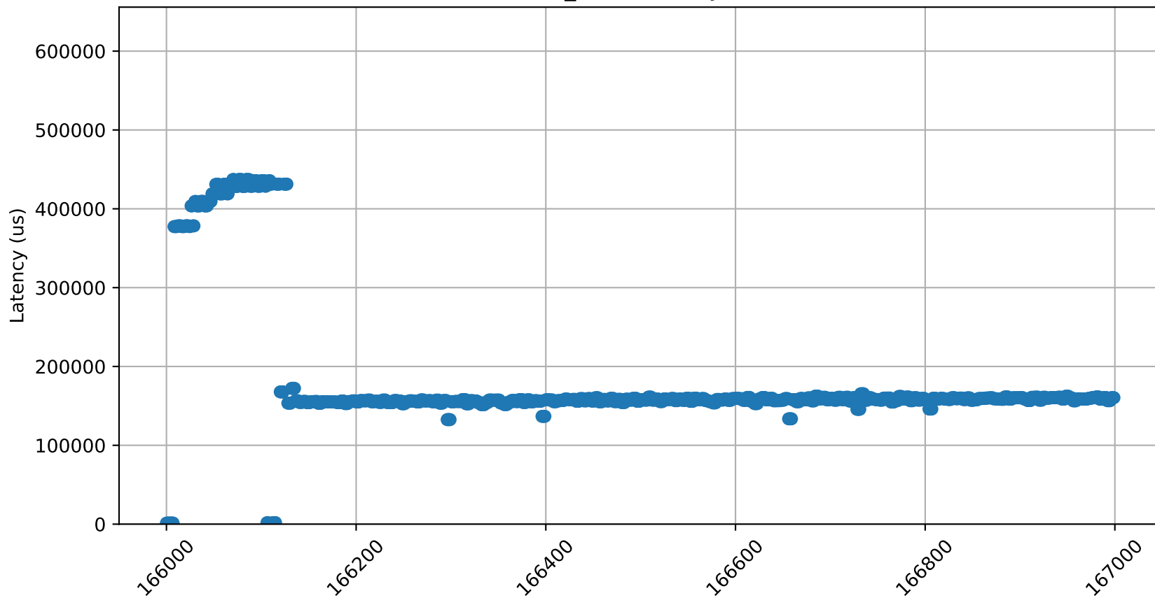
udlB_time Latency(us)
