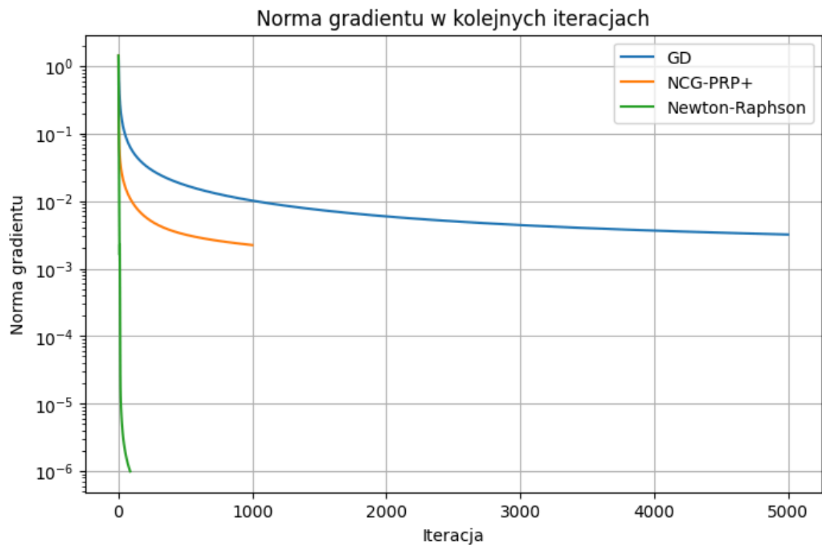
Rysunek 2. Norma gradientu dla metod GD, NCG-PRP+ i Newton-Raphson.
