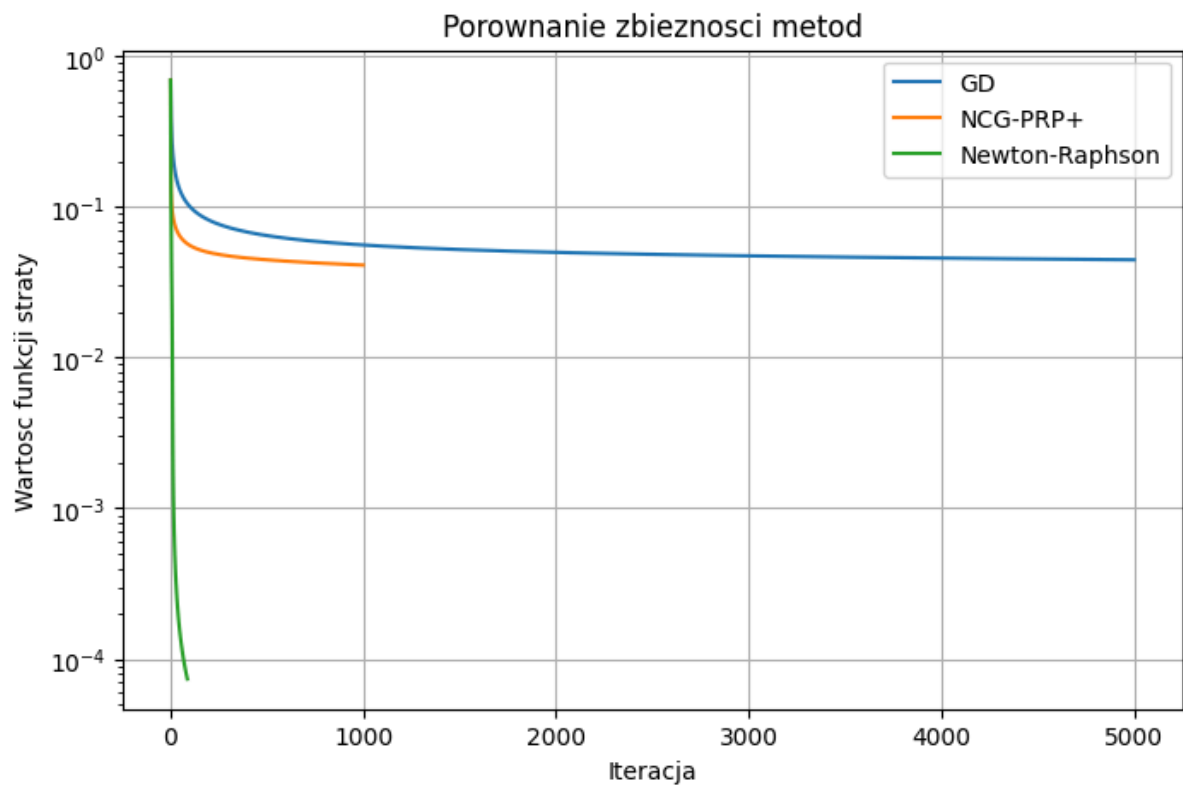
Rysunek 1. Wartość funkcji straty dla metod GD, NCG-PRP+ i Newton-Raphson.
