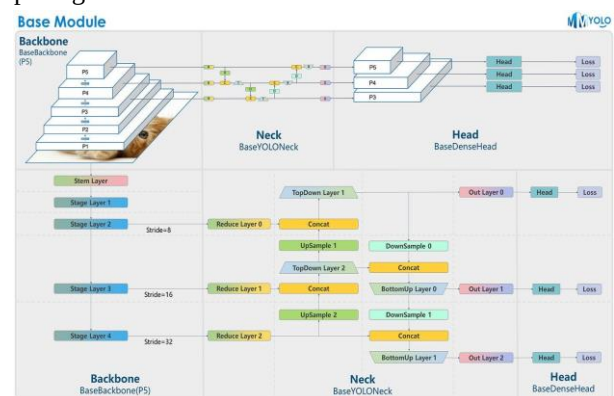
Gambar 1. Arsitektur YOLOv8
