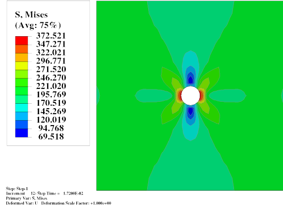
(b) von Mises stress, Frame 2
