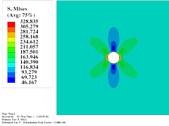
(a) von Mises stress, Frame 1
