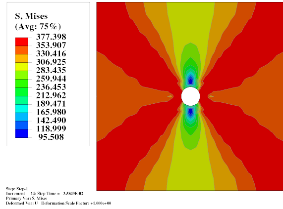
(d) von Mises stress, Frame 4
