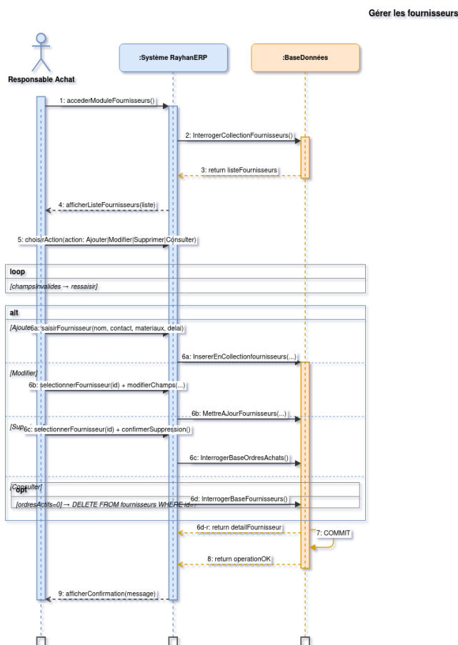
Figure 3.12: Diagramme de séquence : « Gérer Fournisseurs »
