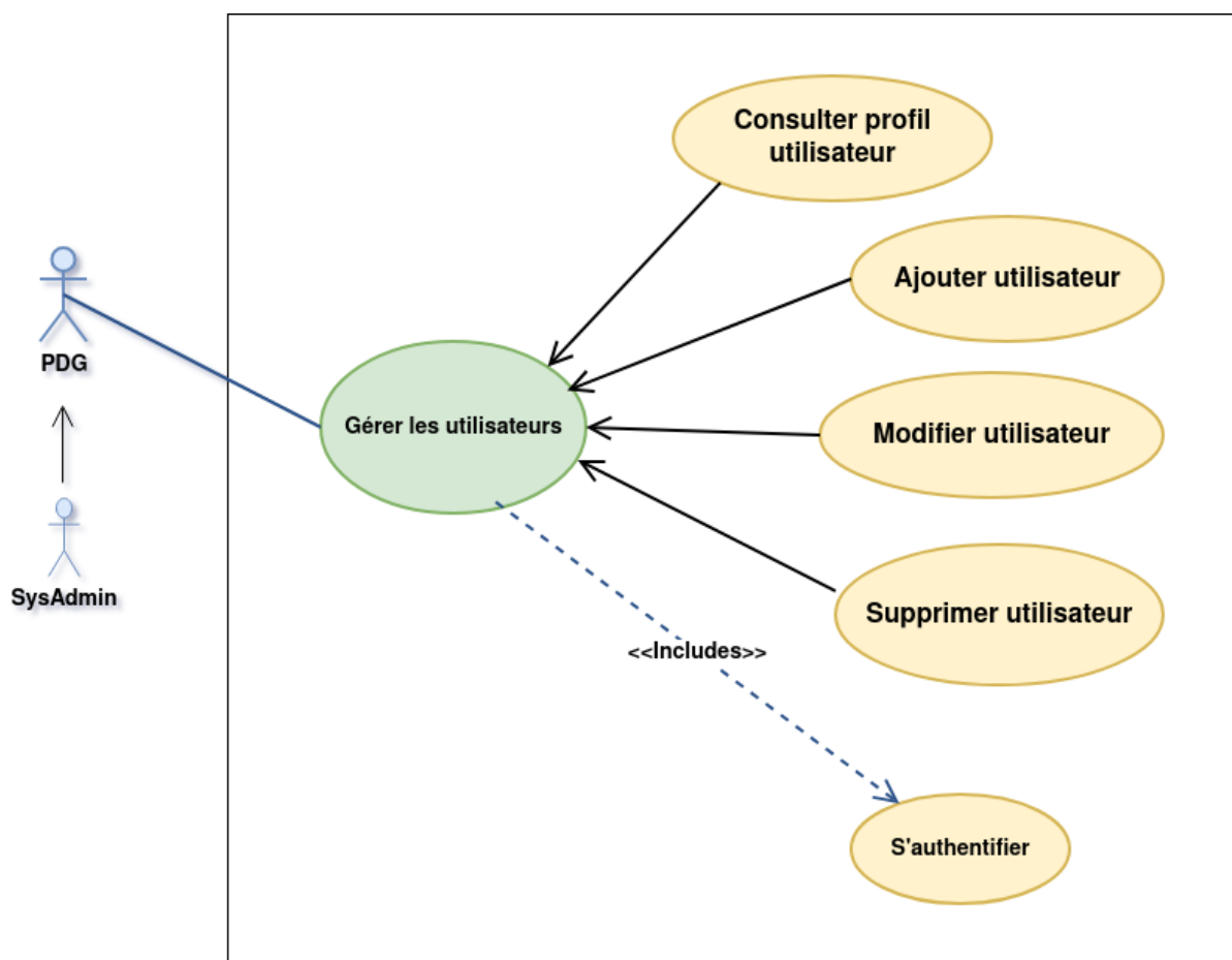
Figure 3.8: Diagramme du cas d'utilisation « gérer les utilisateurs »
