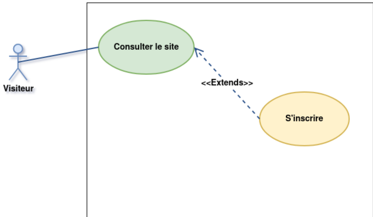
Figure 3.1: Diagramme de cas d'utilisation « Consulter le site »
