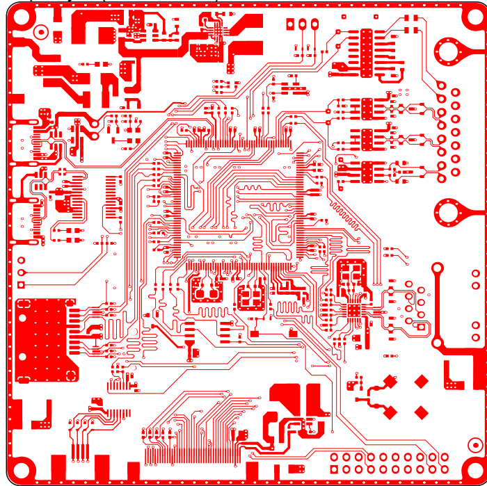
Bottom Layer (Scale 1:1.09)
