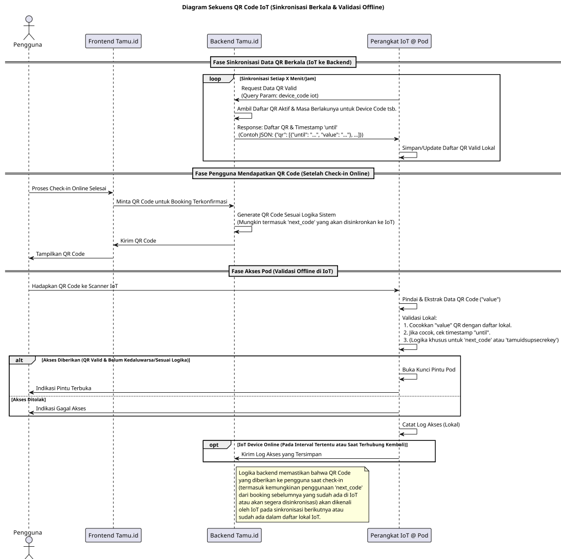
Gambar 3.37 Diagram Sekensial Implementasi Offline Fault Tolerance pada Rotasi Kunci Pod
