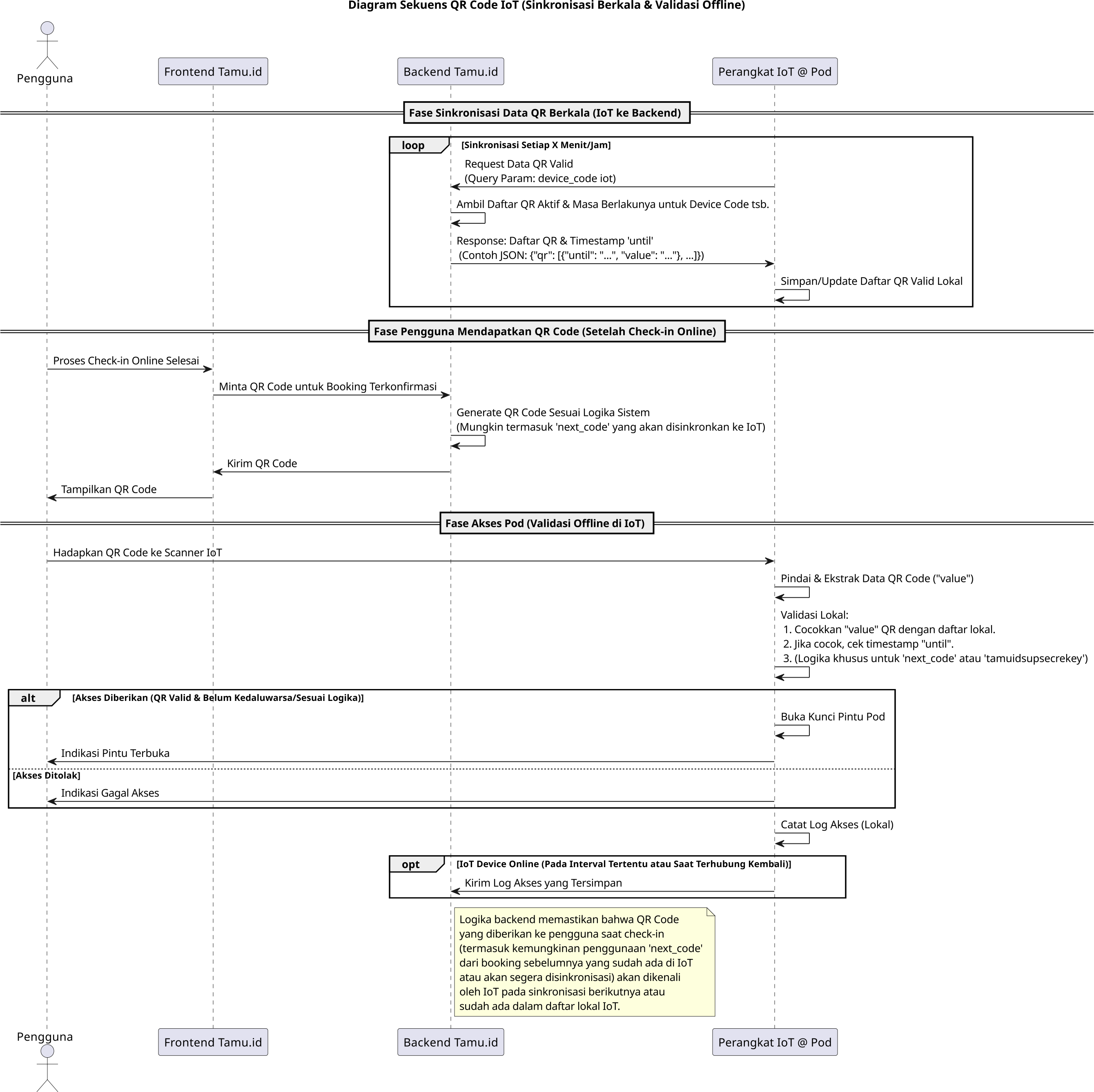
Diagram Sekuens QR Code IoT (Sinkronisasi Berkala & Validasi Offline)
