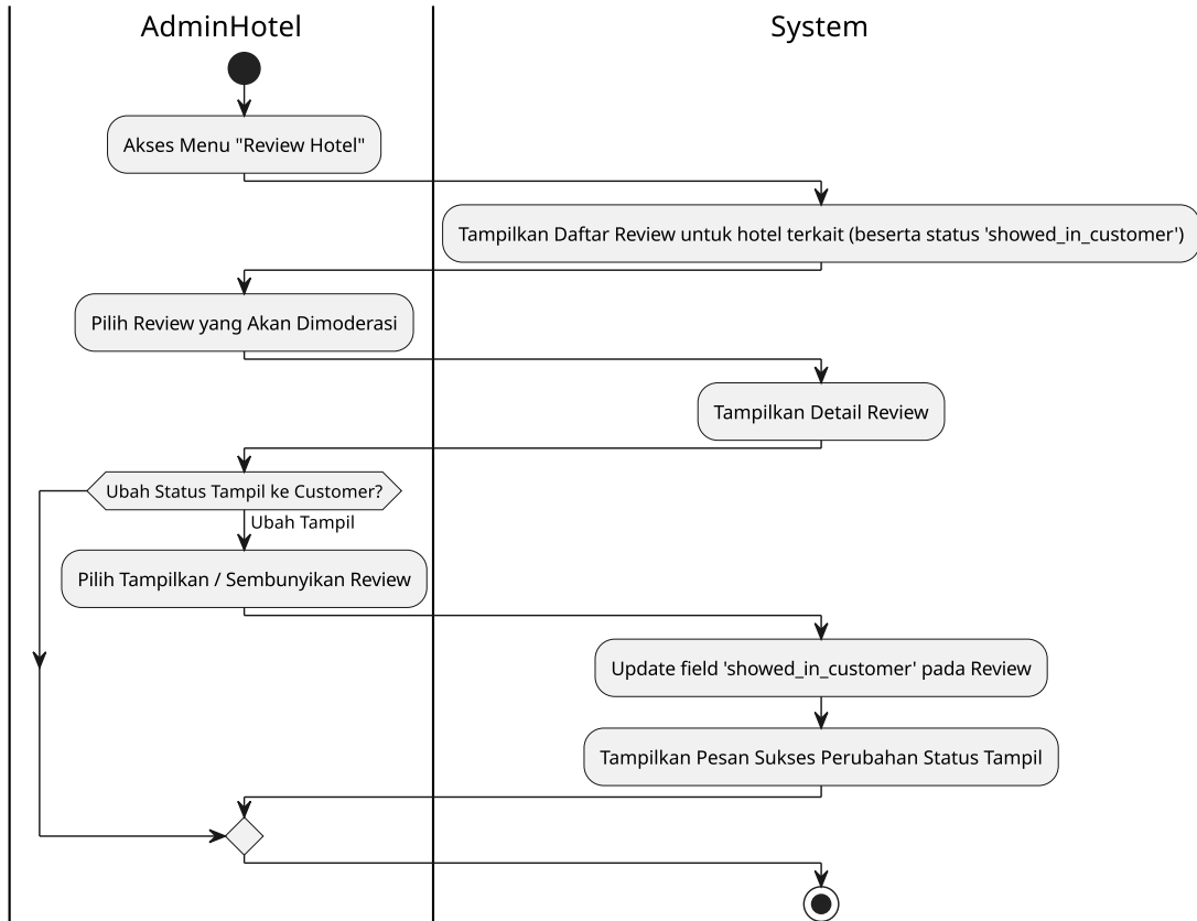
Gambar 3.20 Diagram Aktivitas Admin: Moderasi Review
