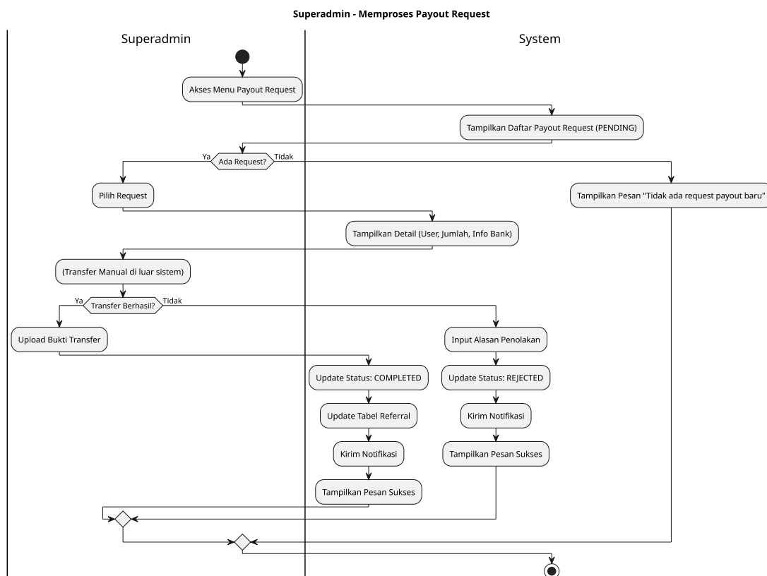
Gambar 4.1 Diagram Aktivitas SuperAdmin: Kelola Payout Request
