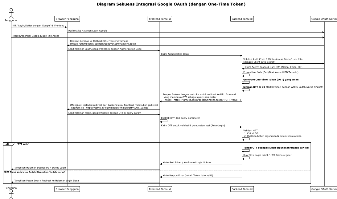
Gambar 3.39 Diagram Sekuensial Integrasi Passwordless dengan OAuth2 Google
