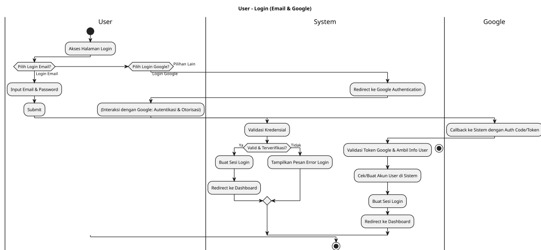
Gambar 3.9 Diagram Aktivitas Pengguna: Registrasi dan Login dengan Google OAuth2
