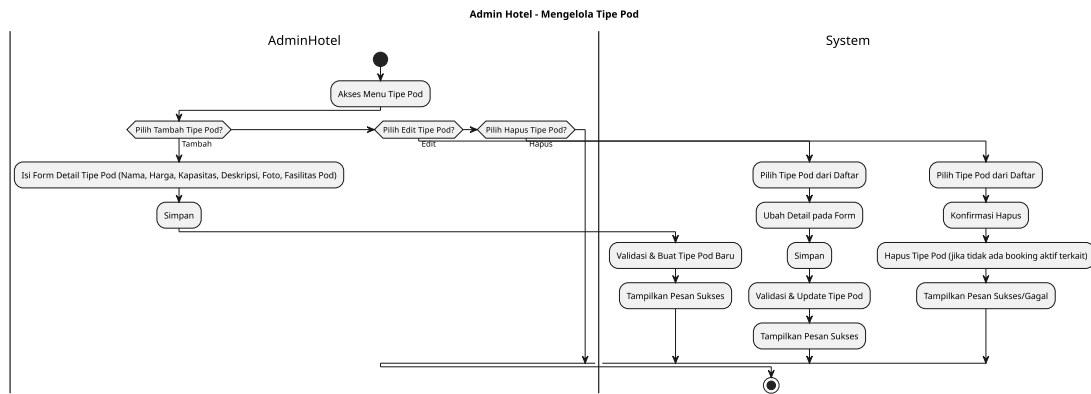
Gambar 3.18 Diagram Aktivitas Admin: Kelola Jenis Pod
