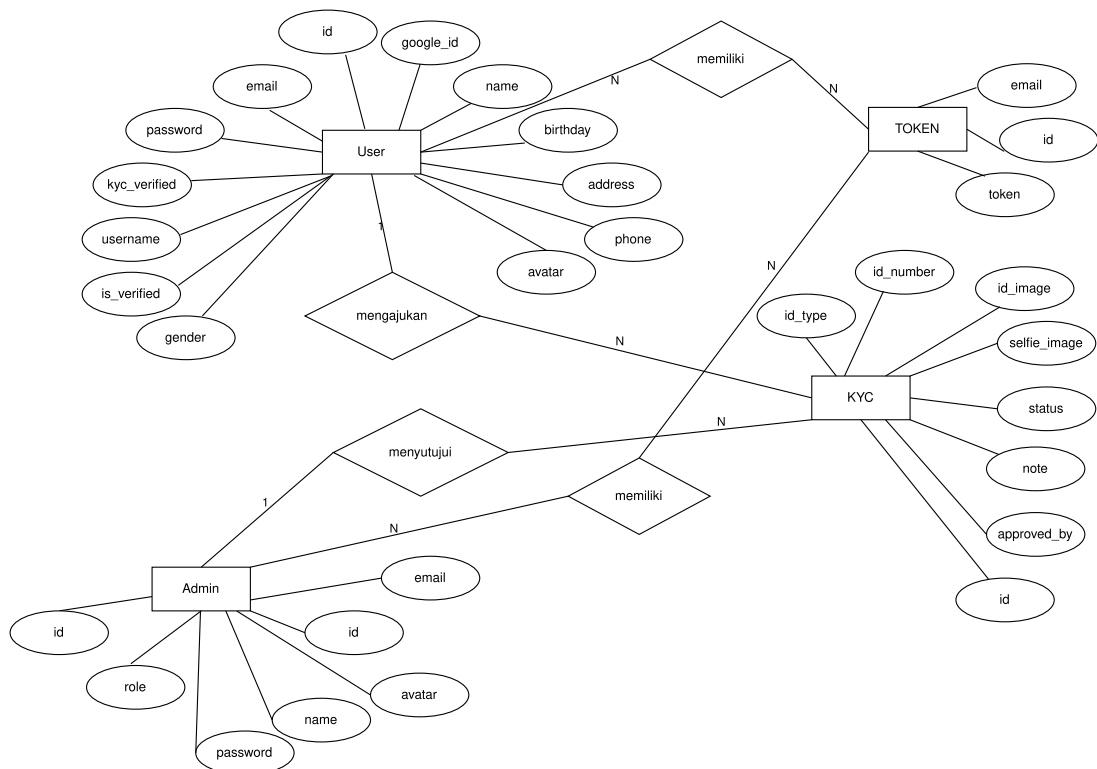
Gambar 3.31 ERD User, Verifikasi Identitas, Admin, dan Token Verifikasi Global
