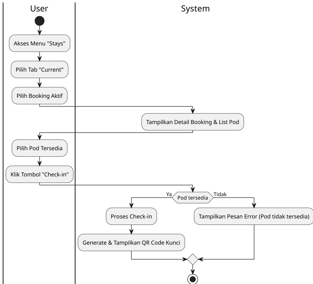
Gambar 3.11 Diagram Aktivitas Pengguna: Checkin dan Stay
