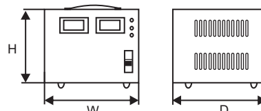
استابلایزر دیجیتال سروو موتوری ایستاده تک فاز
