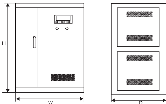
استابلایزر دیجیتال سروو موتوری ایستاده LCD دار سه فاز
