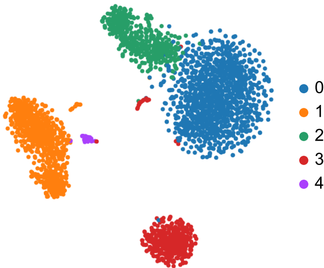
TSNE - leiden_res0.3
