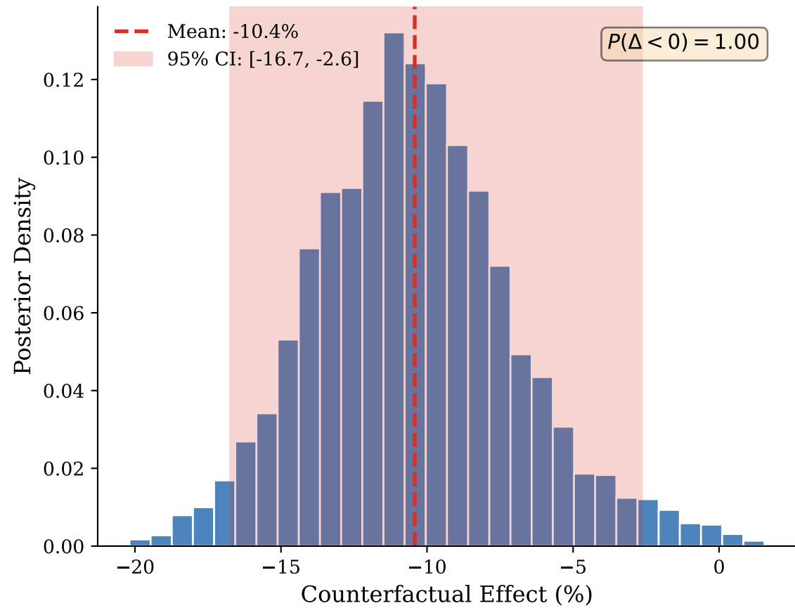
B. Posterior Predictive for Counterfactual
