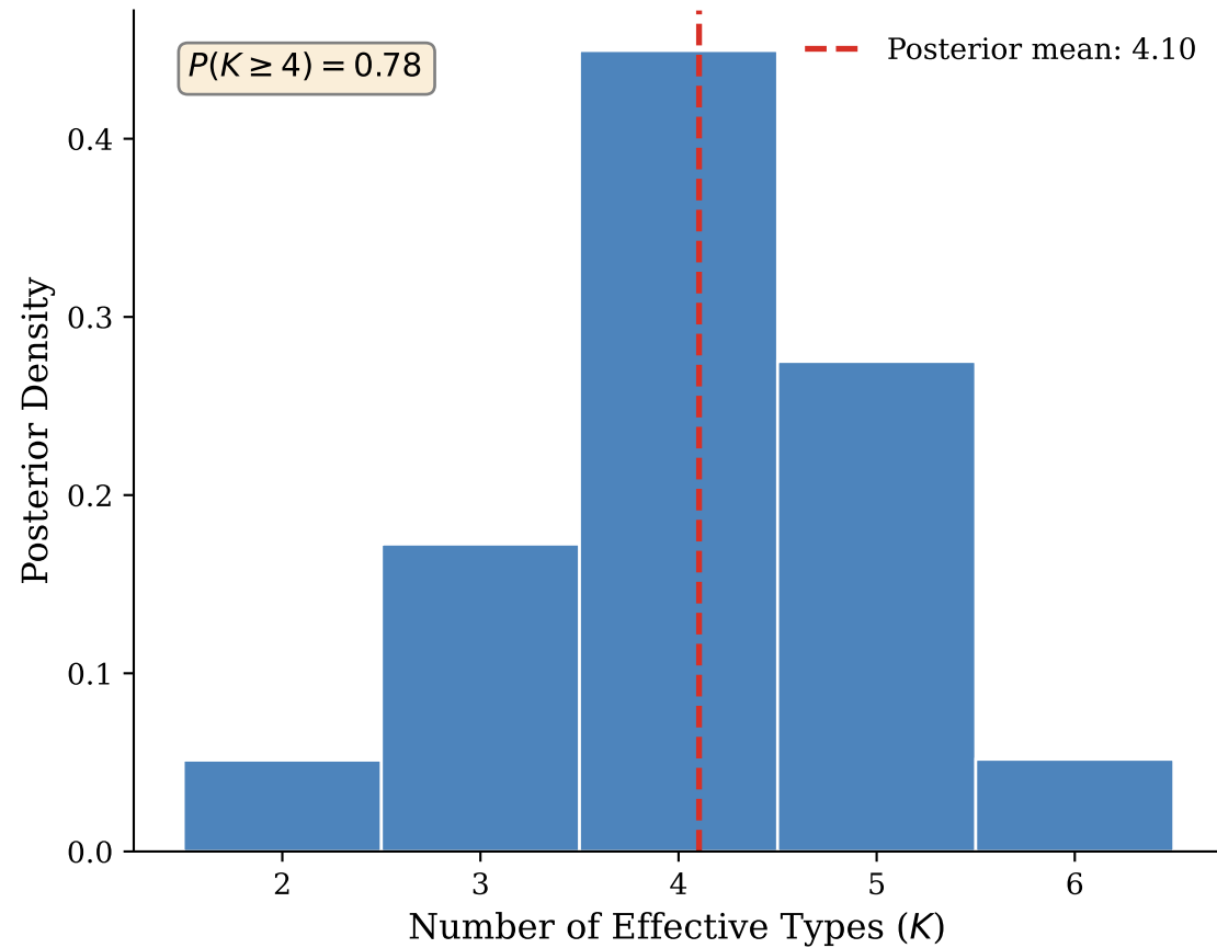
A. Posterior Distribution over K
