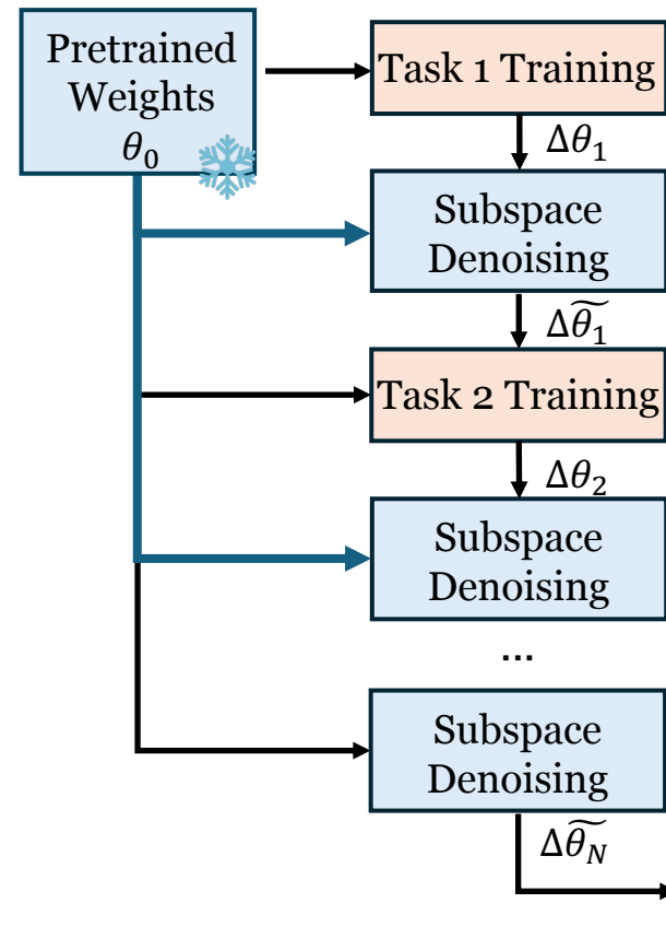
(a) SLoRA-Pre
