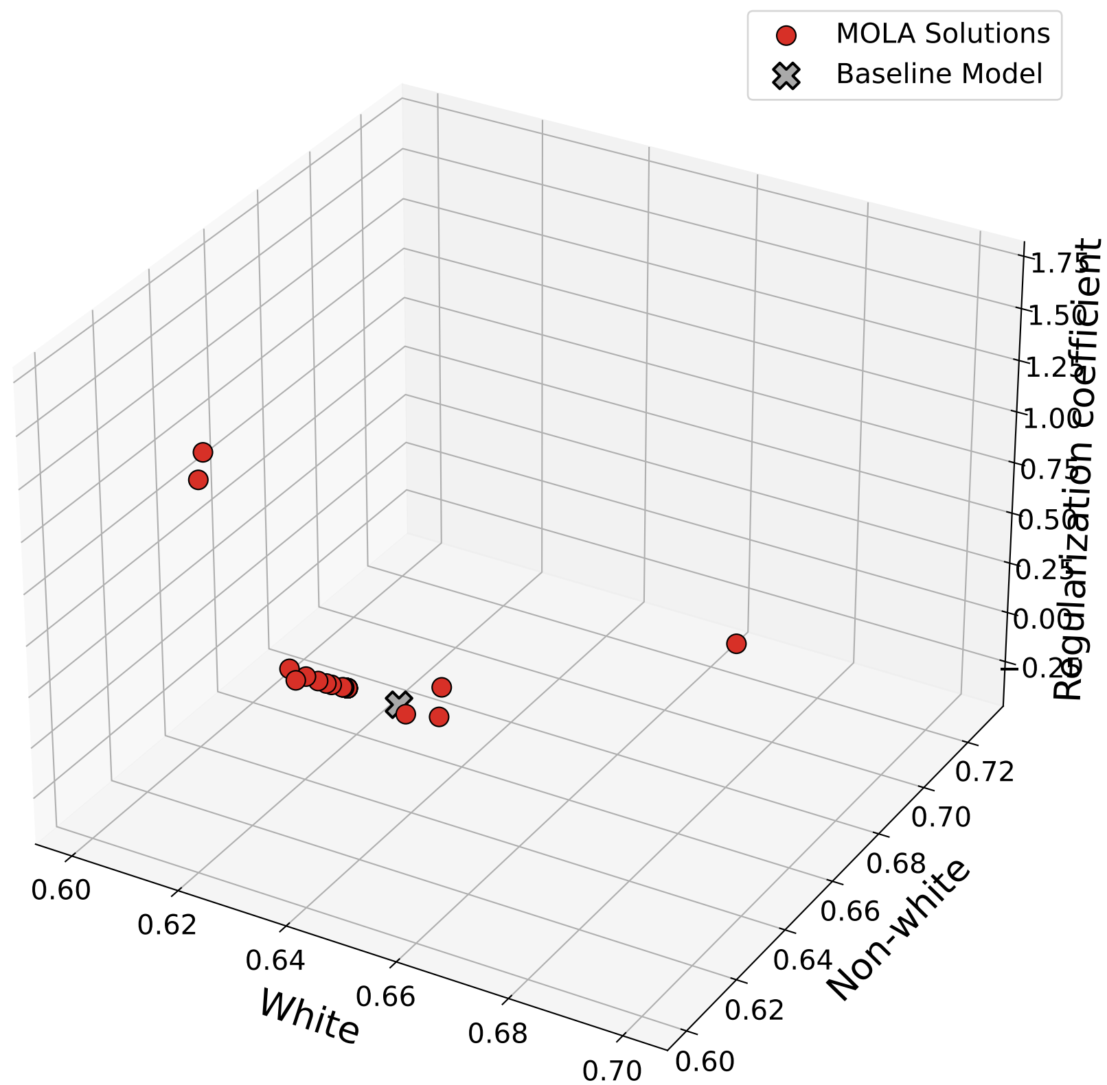
Pareto Frontier
