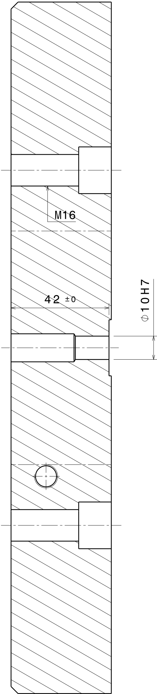
Schnittansicht S-S Maßstab: 1:1
