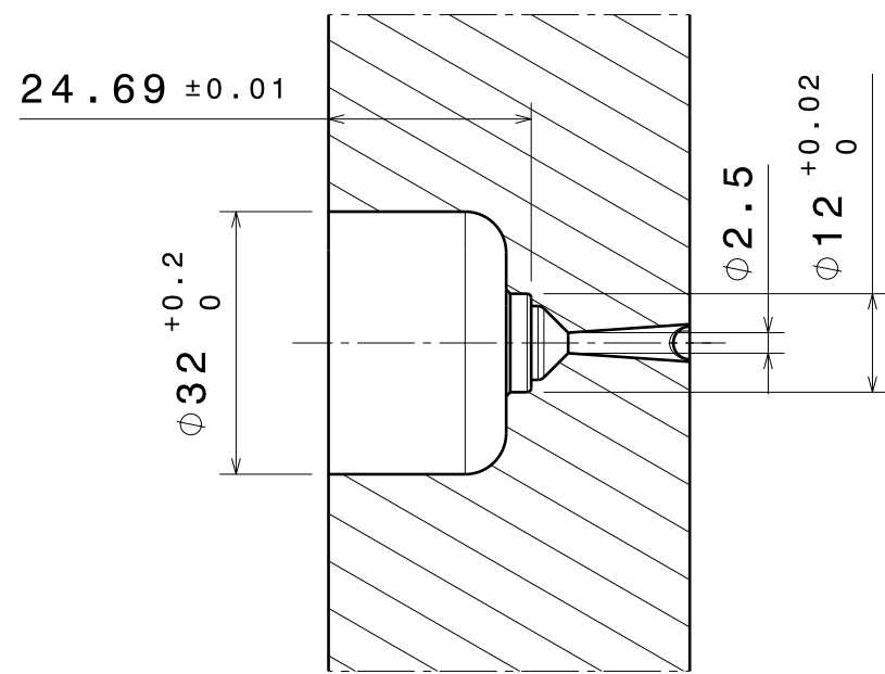
Schnittansicht T-T Maßstab: 1:1
