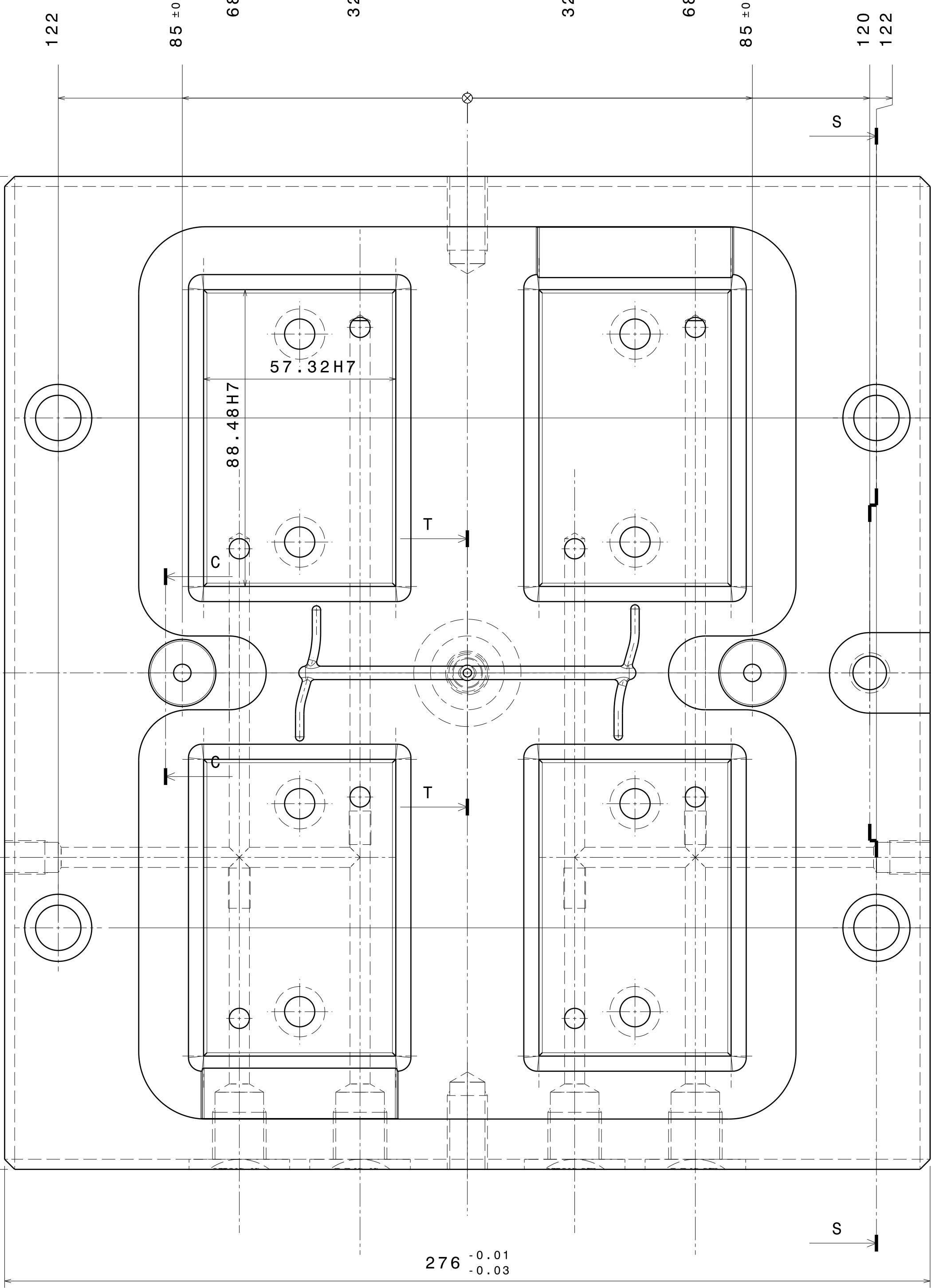
Vorderansicht Maßstab: 1:1
