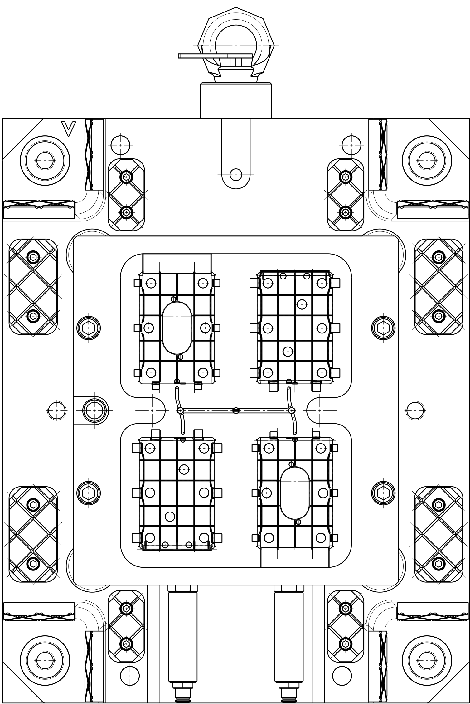
Vorderansicht Maßstab: 1:2
