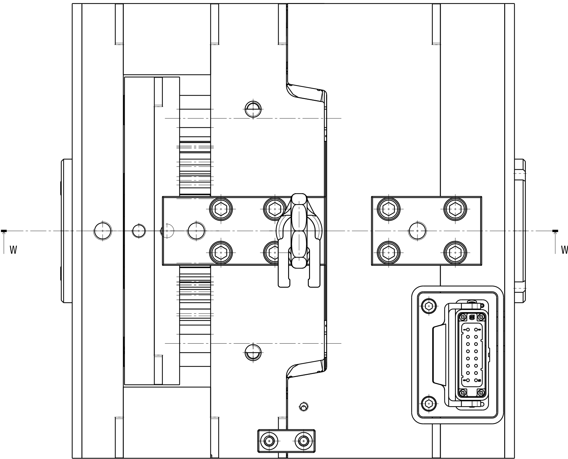
Vorderansicht Maßstab: 1:2
