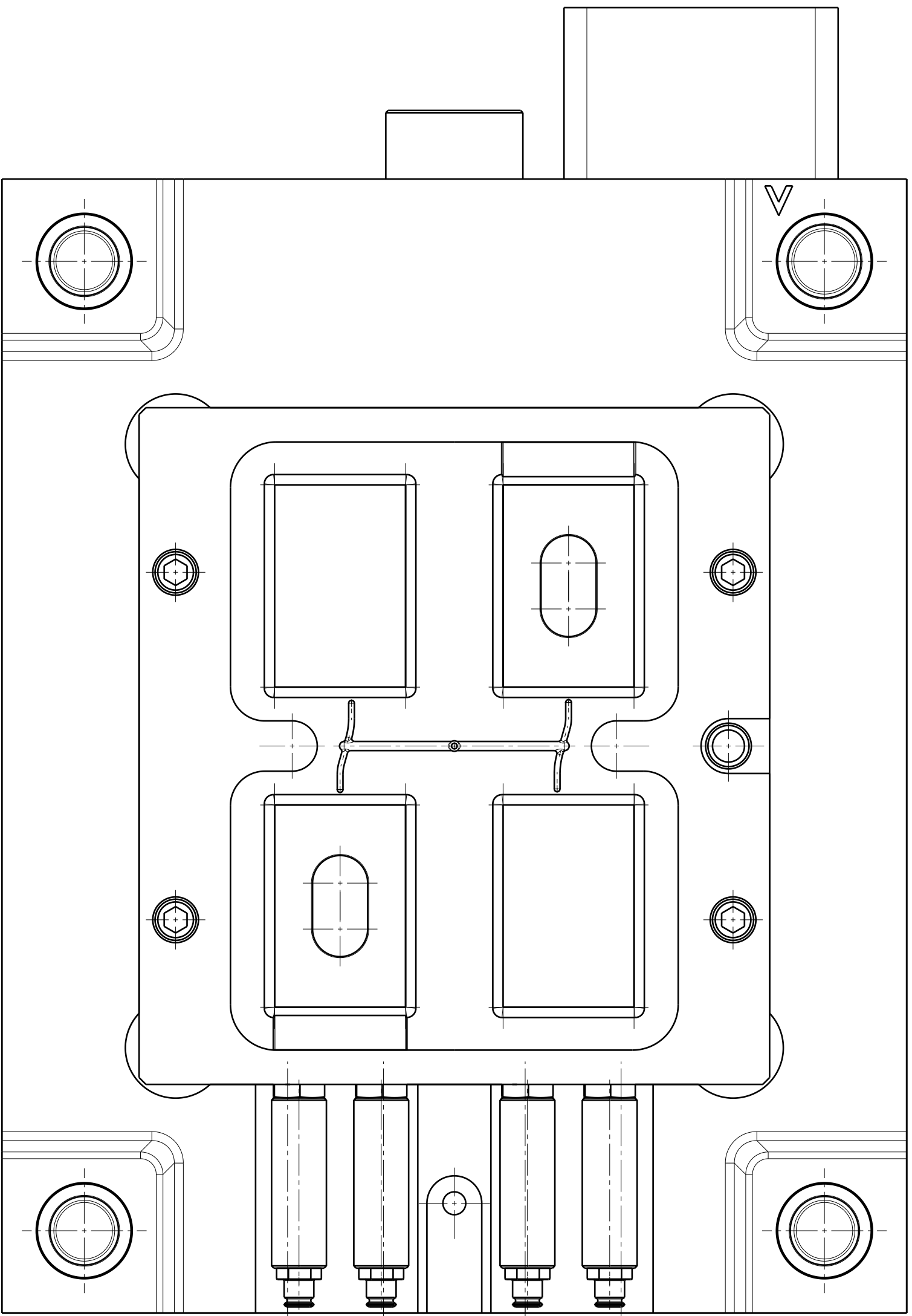
Vorderansicht Maßstab: 1:2
