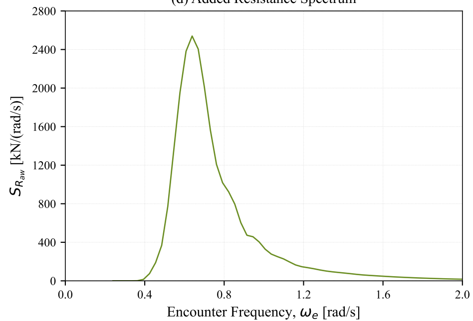
(d) Added Resistance Spectrum
