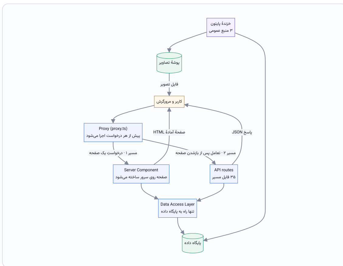
شکل ۴-۱ - معماری کلی سامانه. صرف‌نظر از اینکه درخواست از کدام مسیر بیاید، در نهایت از یک Data Access Layer (لایه واحد دسترسی به داده) رد می‌شود؛ و Proxy پیش از هر چیز روی مسیر قرار دارد.
