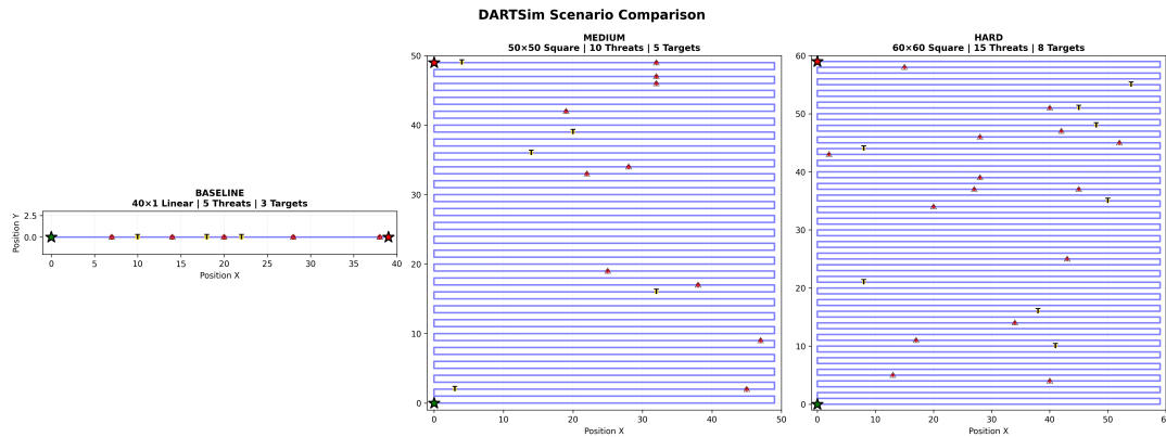
شکل ۲-۴: مقایسه‌ی سه سناریوی DARTSim (پایه، متوسط و سخت)؛ تفاوت در چیدمان نقشه، پیچیدگی مسیر و چگالی تهدید و هدف.
