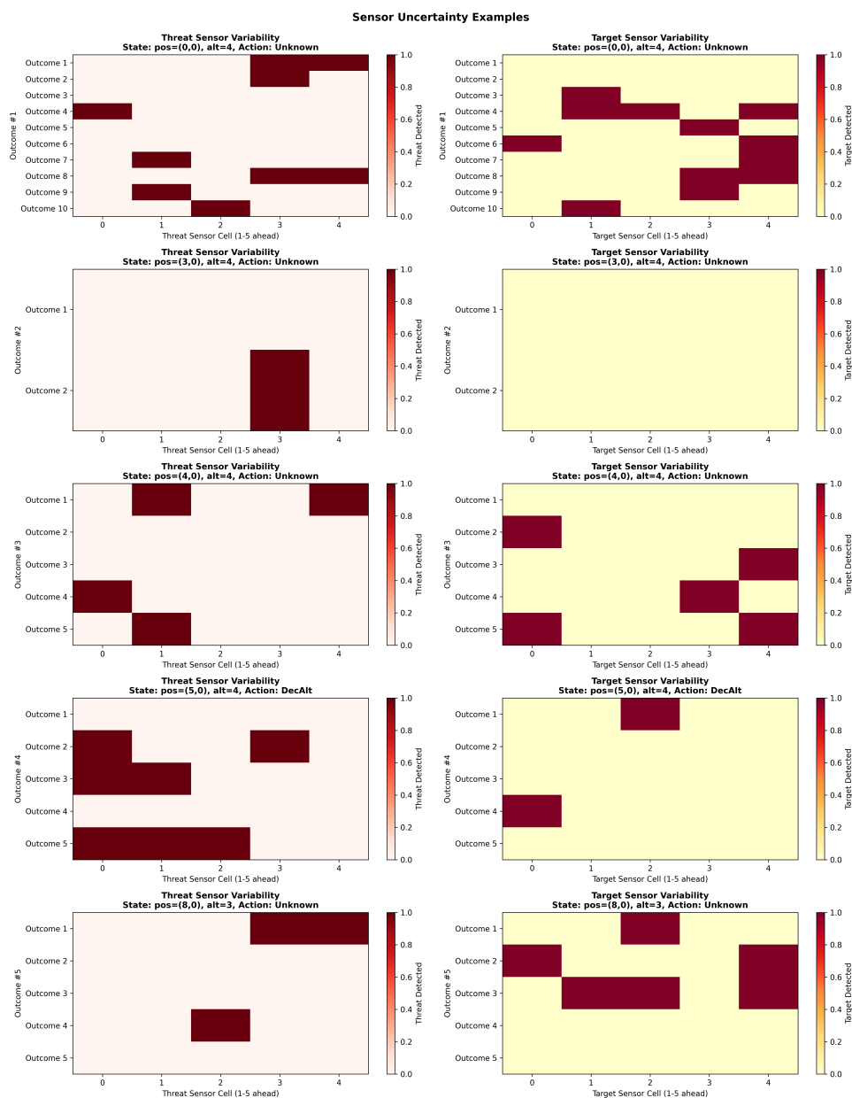
شکل ۲-۳: نمونه‌هایی از تغییرپذیری قرائت حسگرهای تهدید و هدف برای یک زوج حالت-اقدام یکسان در DARTSim؛ هر سطر یک پیامد ممکن و هر ستون یک سلول حسگر پیش‌رو را نشان می‌دهد.
