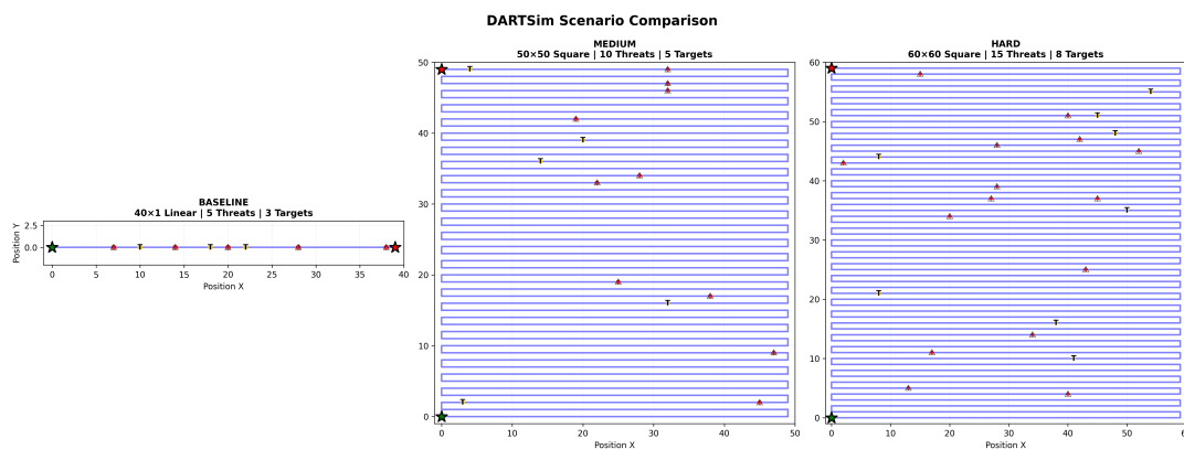
شکل ۲-۵: مقایسه ی سه سناریوی DARTSim (پایه، متوسط و سخت)؛ تفاوت در چیدمان نقشه، پیچیدگی مسیر و چگالی تهدید و هدف.
