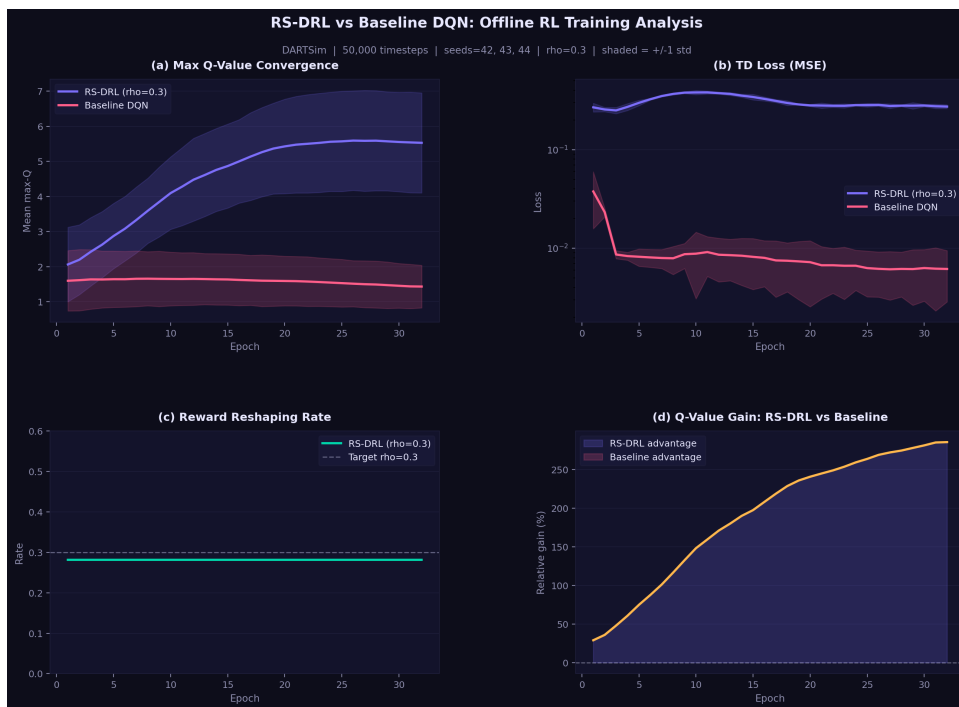
شکل ۵-۴: نمودار همگرایی مأموریت پهبادی DARTSim شامل چهار پانل: (الف) همگرایی ارزش کیو، (ب) میانگین خطای TD، (ج) نرخ شکل دهی پاداش واقعی، و (د) مقایسه گام به گام ارزش کیو.
