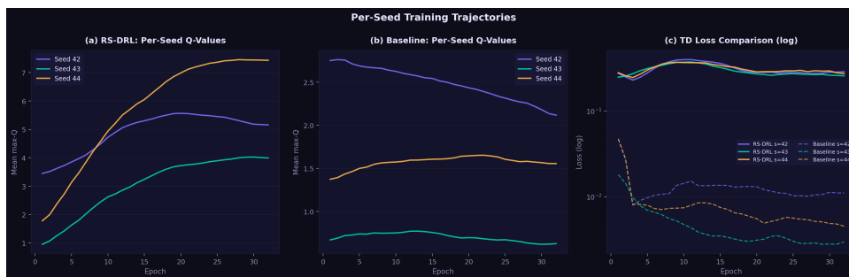
شکل ۵-۵: تحلیل تفکیکی رفتار الگوریتم RS-DRL در مقایسه با DQN پایه به ازای سیدهای تصادفی مستقل ۴۲، ۴۳ و ۴۴ در محیط شبیه ساز پهبادی DARTSim.
