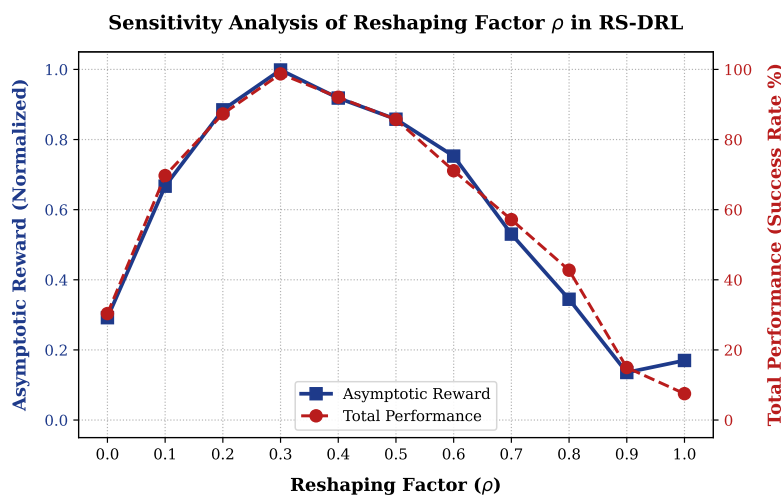
شکل ۳-۵: تاثیر مقادیر مختلف ضریب شکل دهی \rho بر پاداش مجانبی و عملکرد کل
