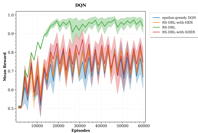
شکل ۵-۲: منحنی‌های یادگیری الگوریتم‌ها در محیط DeltaIoTv1.1
