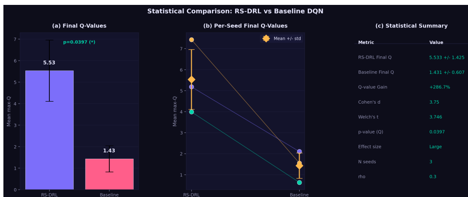
شکل ۵-۶: تحلیل آماری و معناداری اندازه اثر کوهن (Cohen's d) و فواصل اطمینان ارزش کیو برای روش پیشنهادی در برابر روش پایه در مأموریت های DARTSim.
