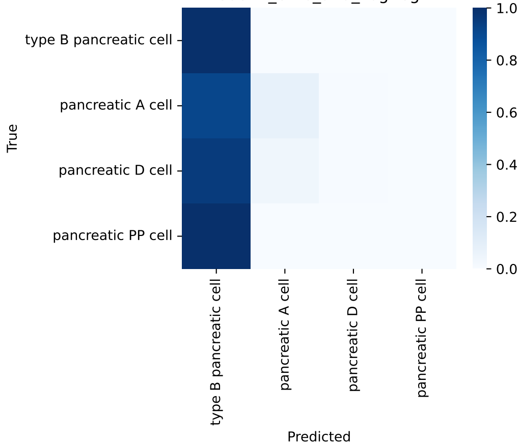
scGPT_emb_and_LogReg
