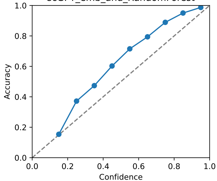
scGPT_emb_and_RandomForest
