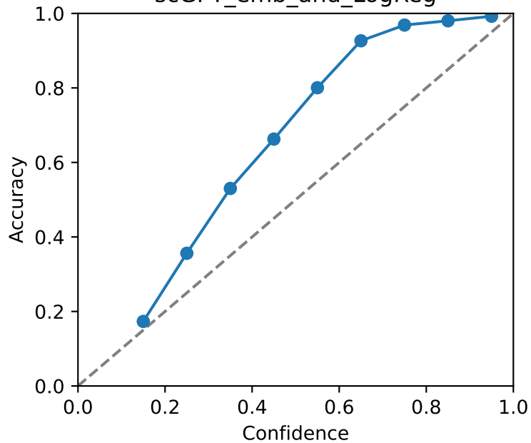
scGPT_emb_and_LogReg
