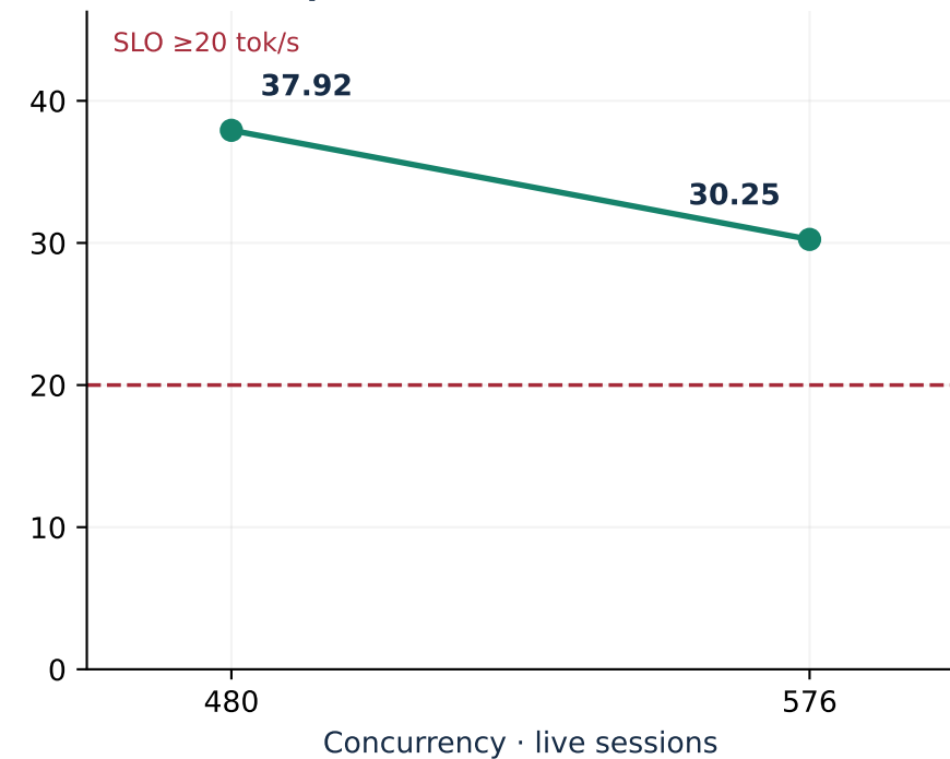
E2E I90 (output tok/s/user)
