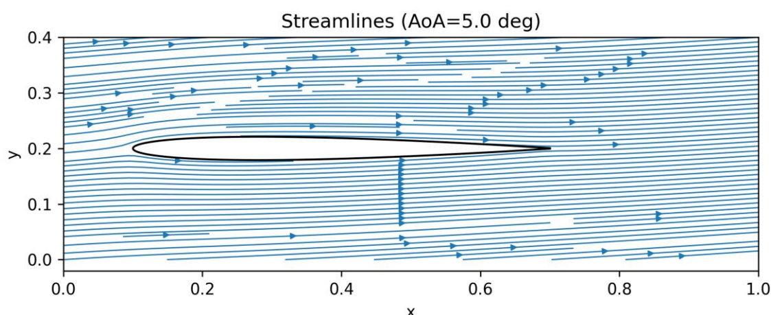
شکل 3.7.3 خطوط جریان حول ایرفویل در زاویه حمله 5
