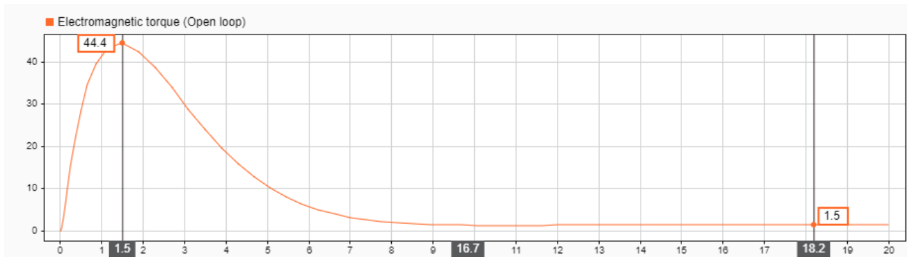
شکل 6 پاسخ گشتاور الکترومغناطیسی موتور در حالت حلقه باز
