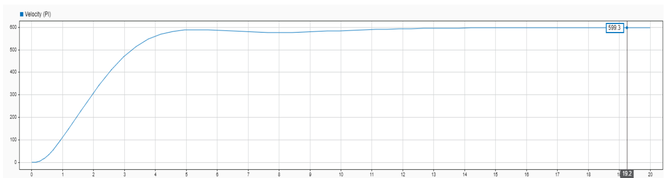
شکل 10 پاسخ سرعت موتور با کنترلر PI
