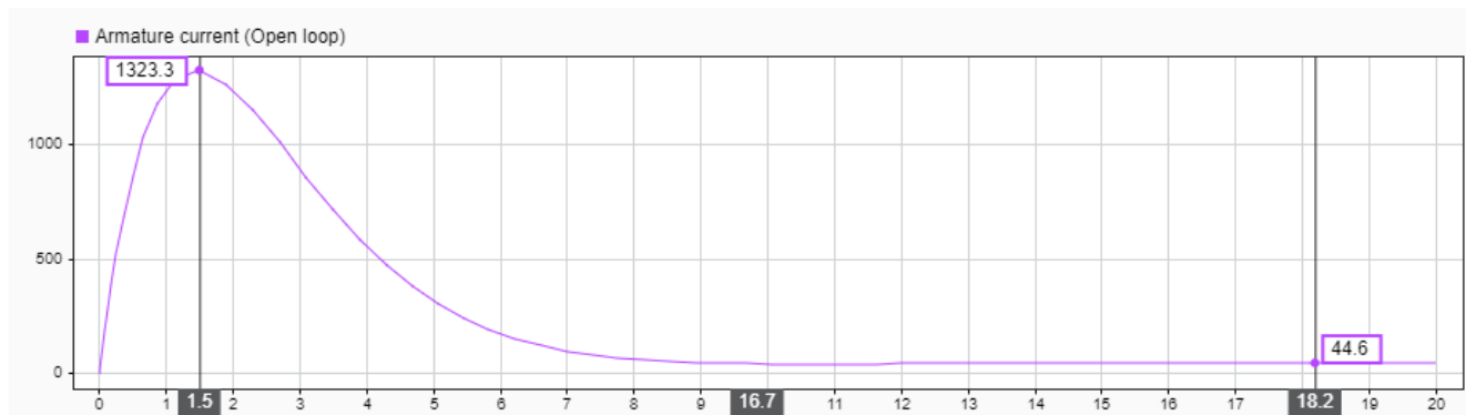
شکل 5 پاسخ جریان آرمیچر موتور در حالت حلقه باز
