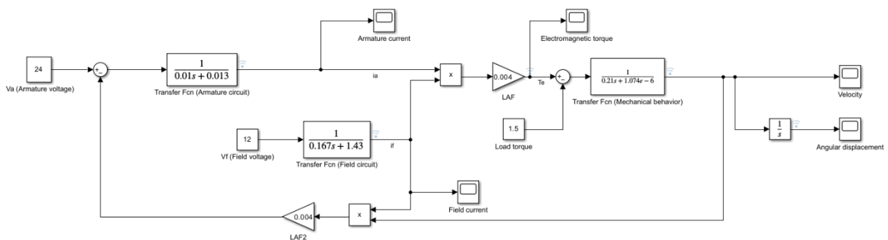
شکل 1 مدل حلقه باز موتور DC تحریک جداگانه تحت بار گشتاور ثابت
