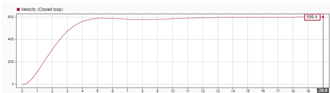
شکل 12 پاسخ سرعت موتور در حالت حلقه بسته
