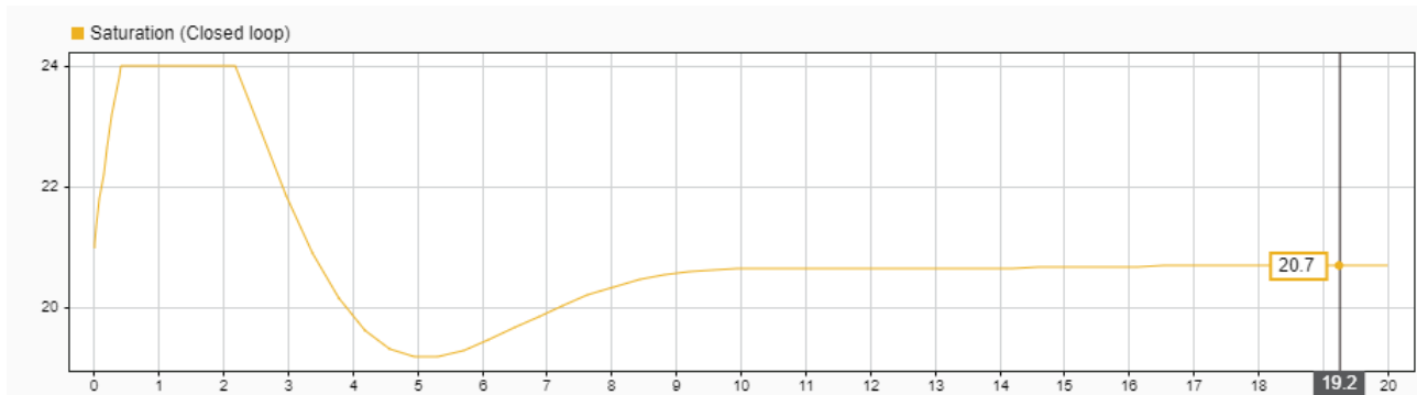
شکل 13 ولتاژ آرمیچر در حالت حلقه بسته
