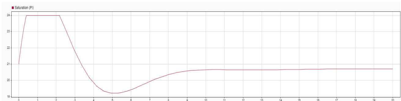
شکل 11 خروجی کنترلر بلوک Saturation در کنترلر PI
