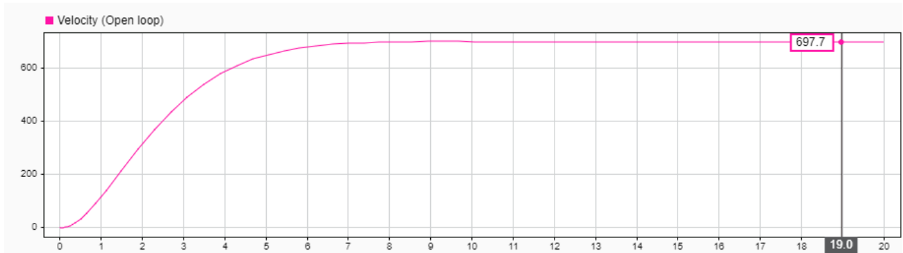
شکل 3 پاسخ سرعت موتور در حالت حلقه باز
