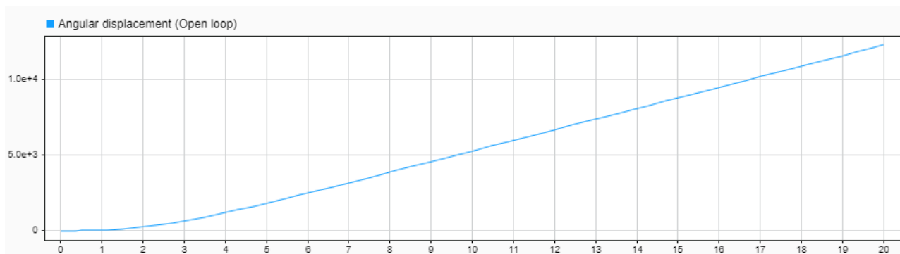
شکل 7 پاسخ جابجایی زاویه‌ای موتور در حالت حلقه باز
