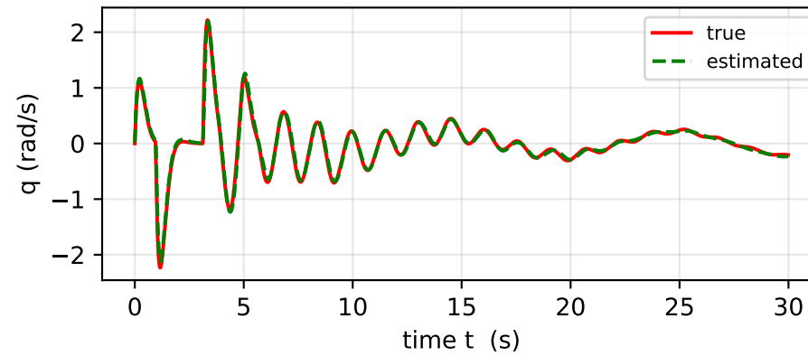
q (HID) RMSE=0.049 rad/s
