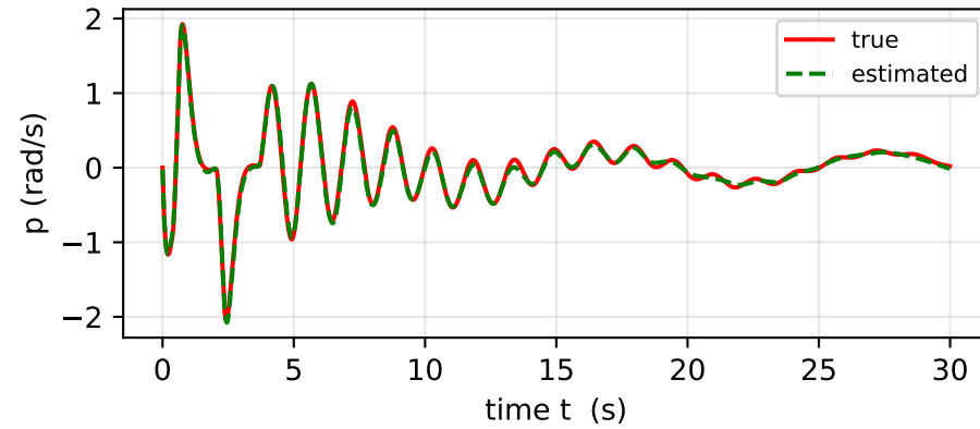
p (HID) RMSE=0.036 rad/s
