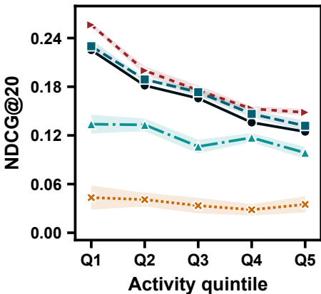
ML-1M
