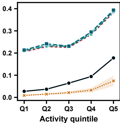
Last.FM
