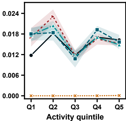
Amazon-VG
