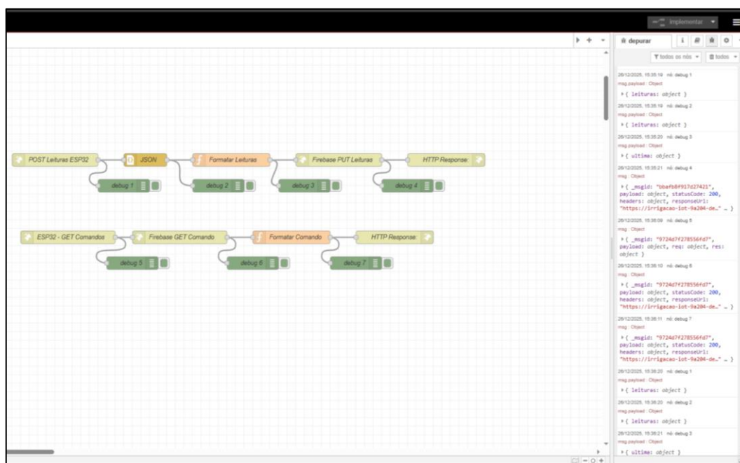
Figura 3 - Configuração da camada de Fog utilizando o Node-RED.
