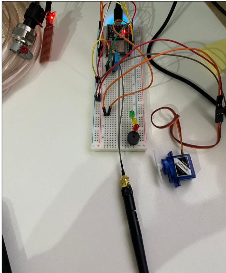
Figura 1 - Componentes eletrônicos utilizados para o desenvolvimento do sistema.
