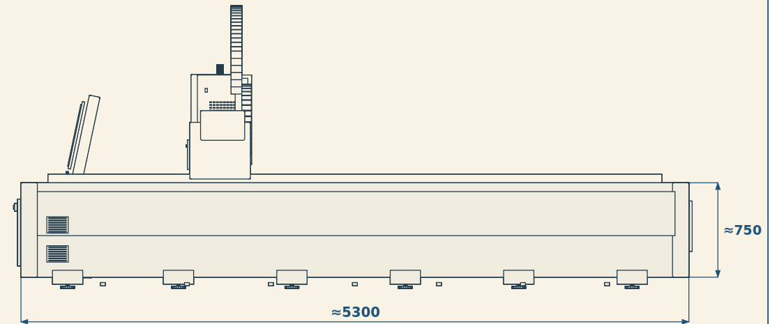
نمای جانبی
