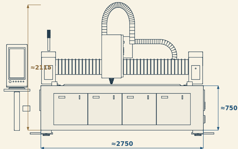
نمای جلو
