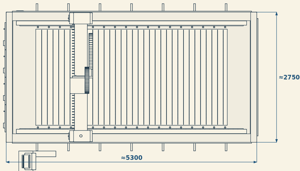
نمای بالا
