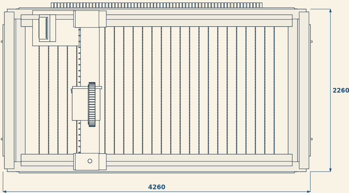
نمای بالا
