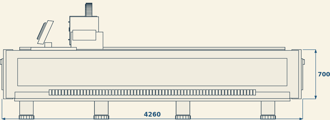
نمای جانبی
